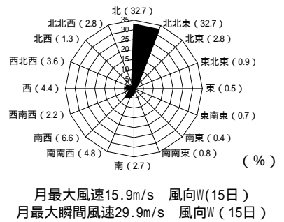
風向別頻度
