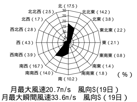
風向別頻度
