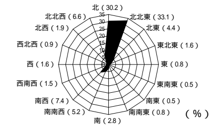
風向別頻度
