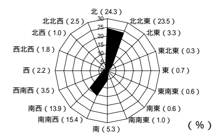
風向別頻度
